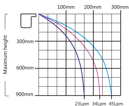
PROYECCIÓN APROXIMADA DE LÁMINA DE AGUA POR 300MM DE LA ALTURA DE LA CASCADA
